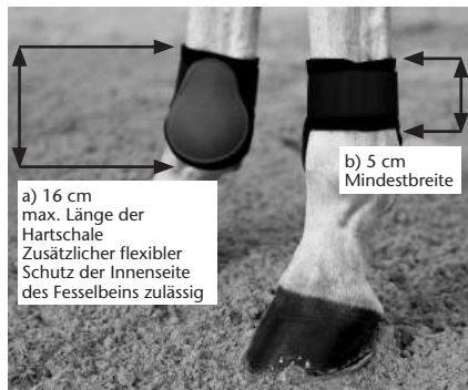
Abb. 22: Streichkappen
